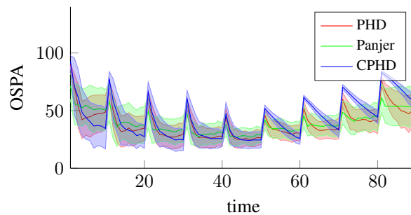
(d) OSPA results, experiment 2.2.
